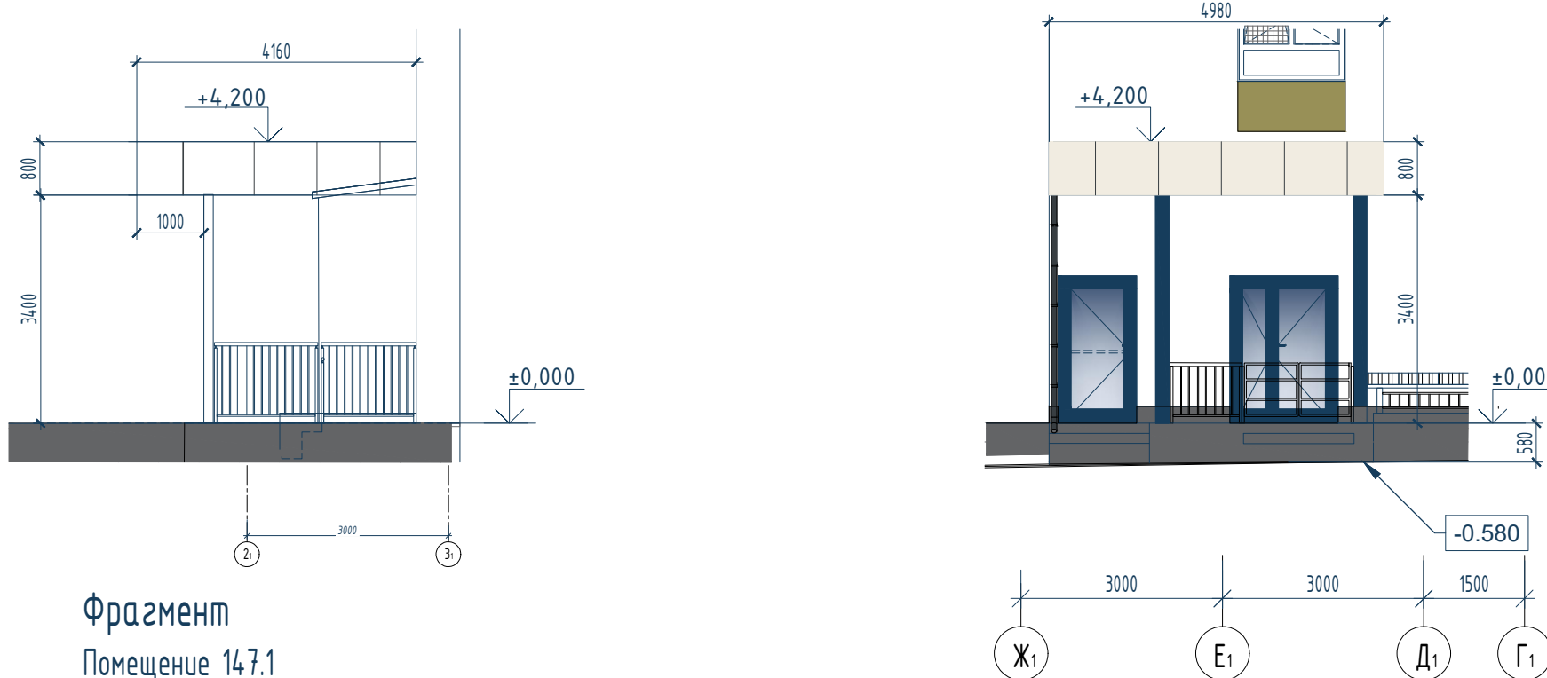
Фрагмент Габаритный размеры и высоты козырька
