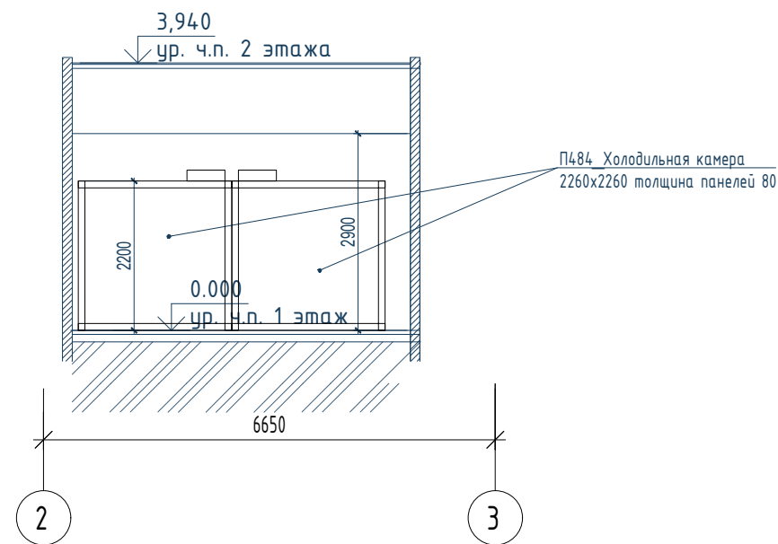
Фрагмент Помещение 147.1 с холодильным оборудованием разрез 1-1
