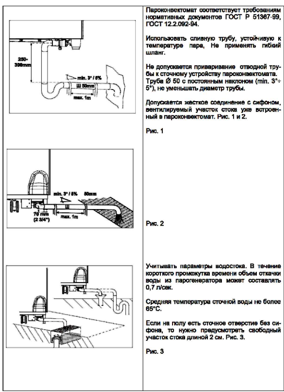
Схема 2 Отвод сточных вод от пароконвектомата
